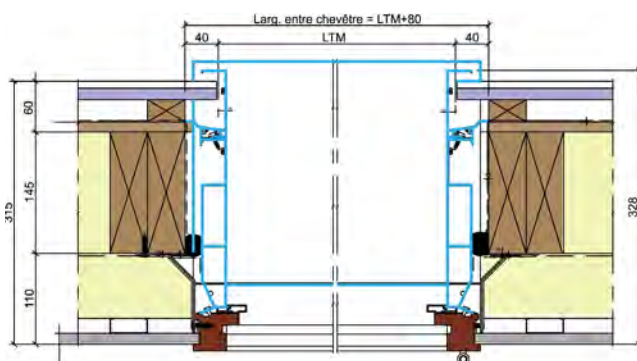
COUPE HORIZONTALE
