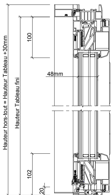
coupe verticale
