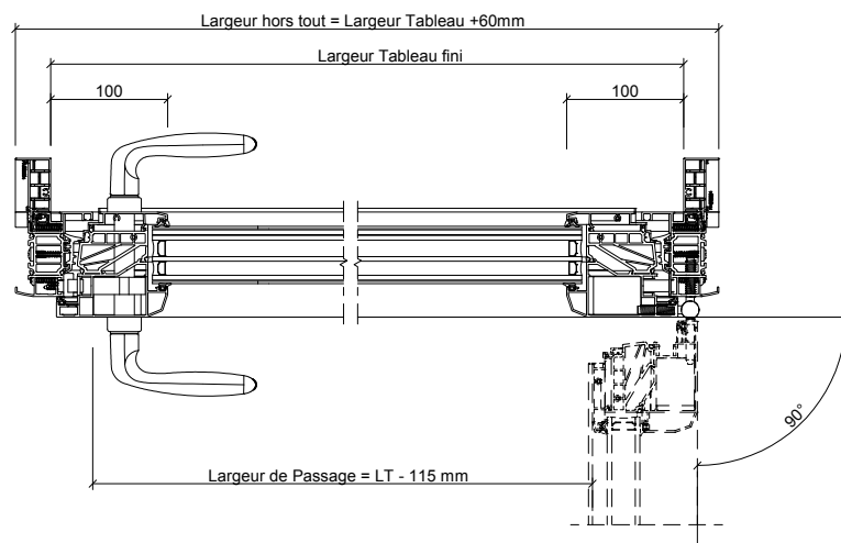
coupe horizontale
